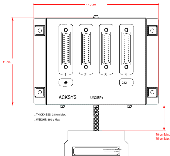
UNXBP 232 4 VOIES
