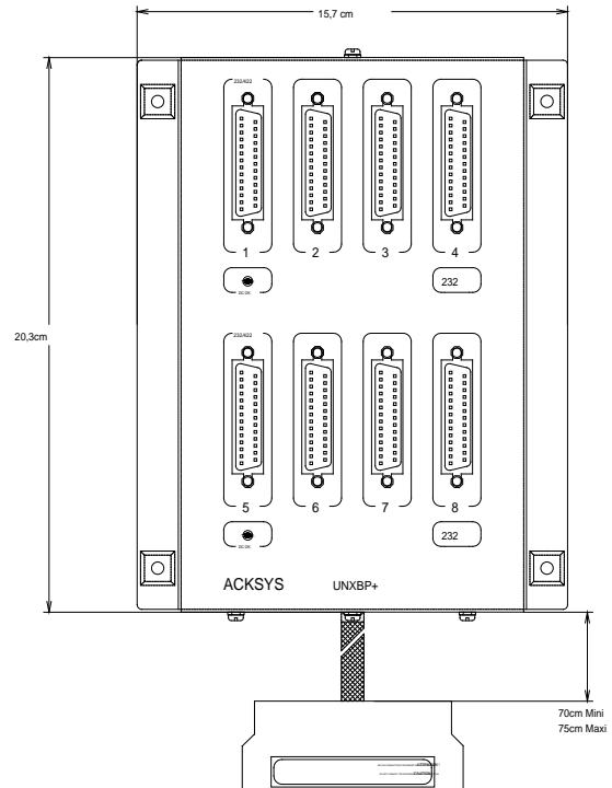
UNXBP 232 8 VOIES
